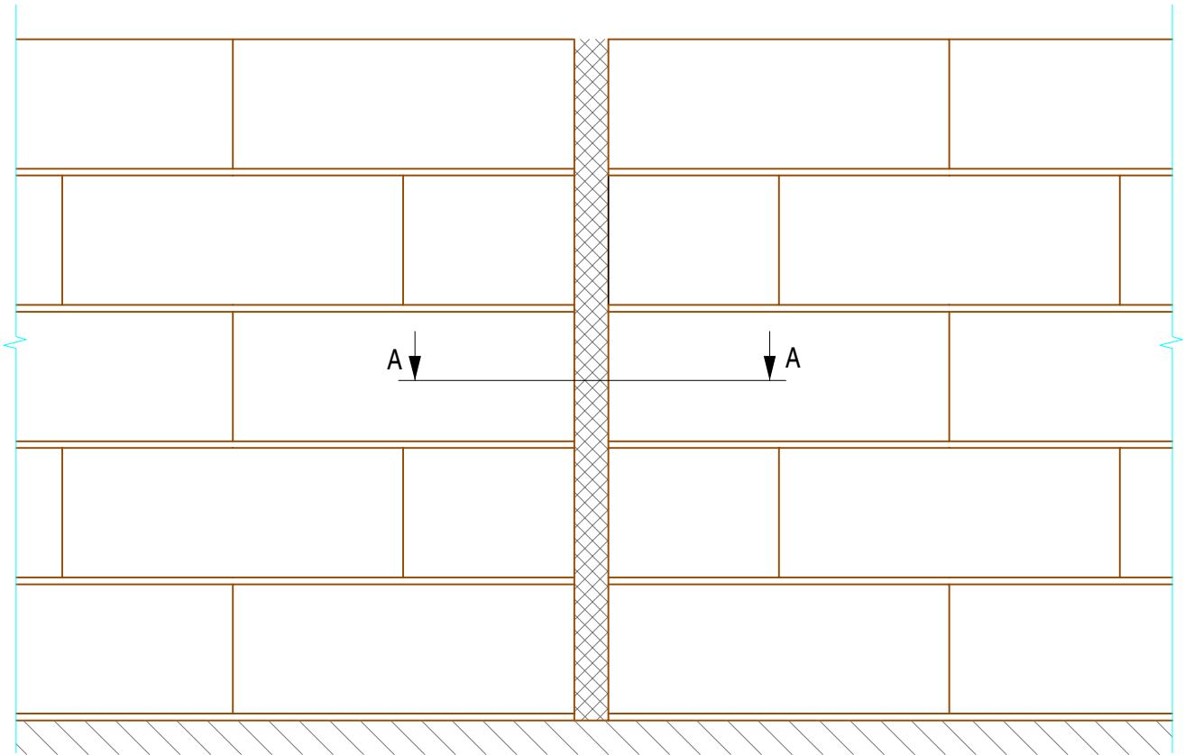
Pjūvis A-A/I var.
