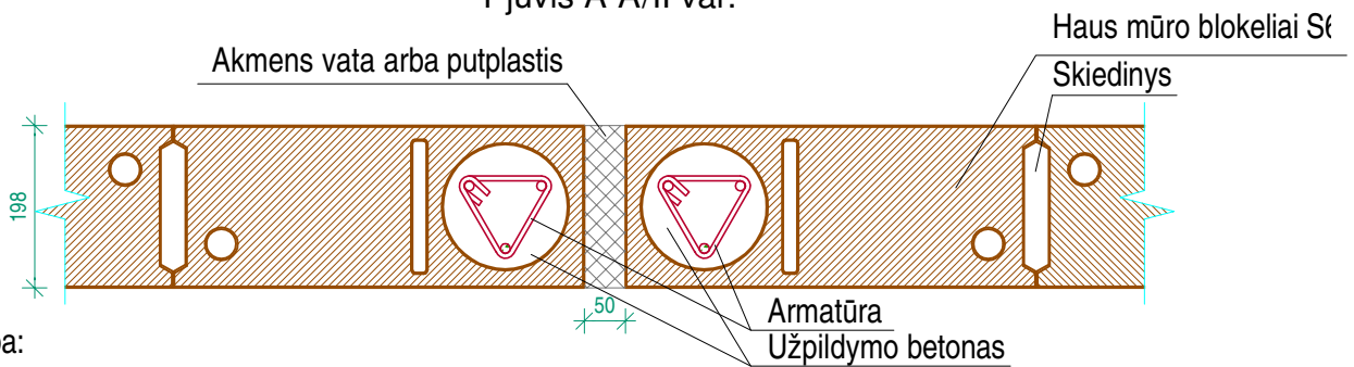
Pjūvis A-A/II var.
