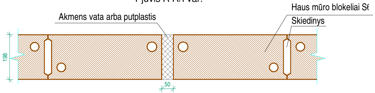
Pjūvis A-A/II var.
